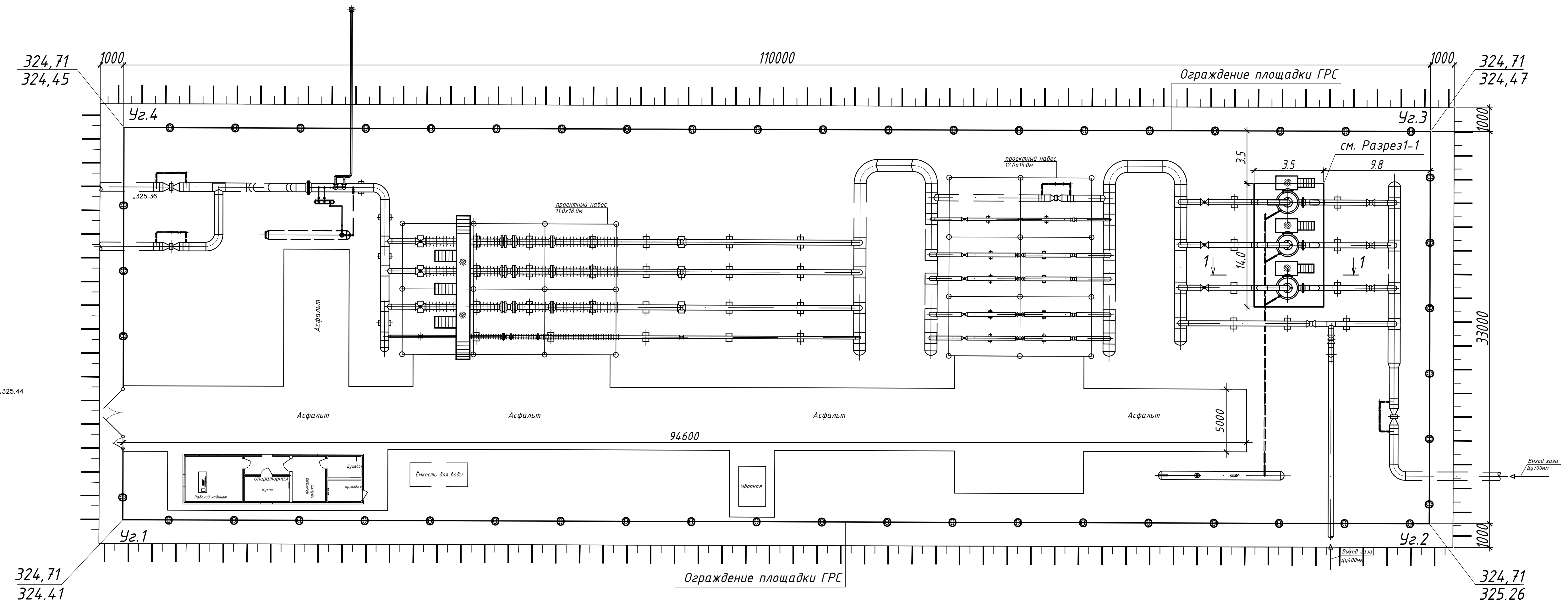
Разбивочный план площадки ГРС М1:500
